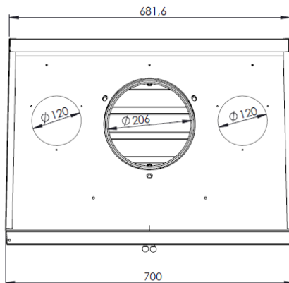
Figura n o 1 - Dimensiones en mm del aparato MIDI-700
