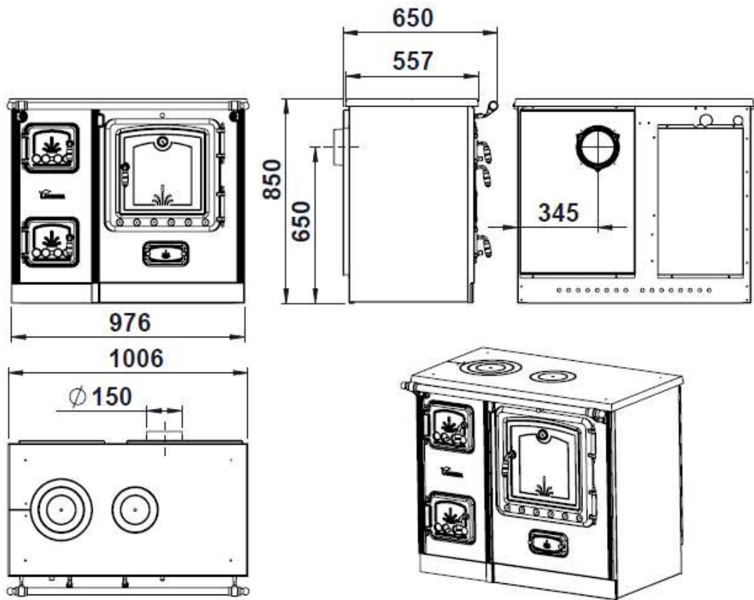
Figura n°3 - Dimensiones en mm del aparato Lis 8T
